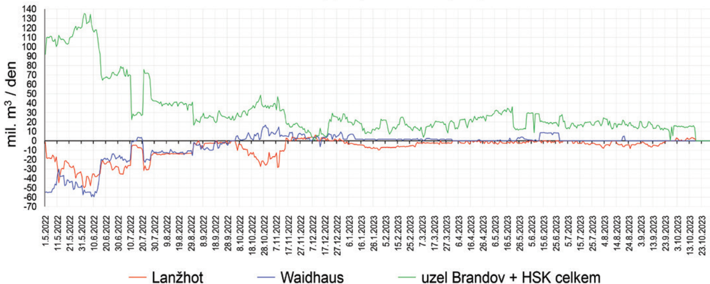
Obr. 4 Změna charakteru toků plynu přes hraniční profily
